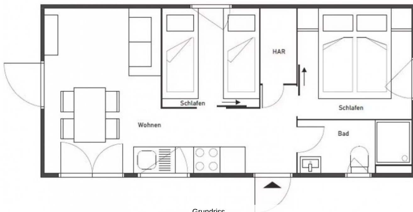
Grundriss
